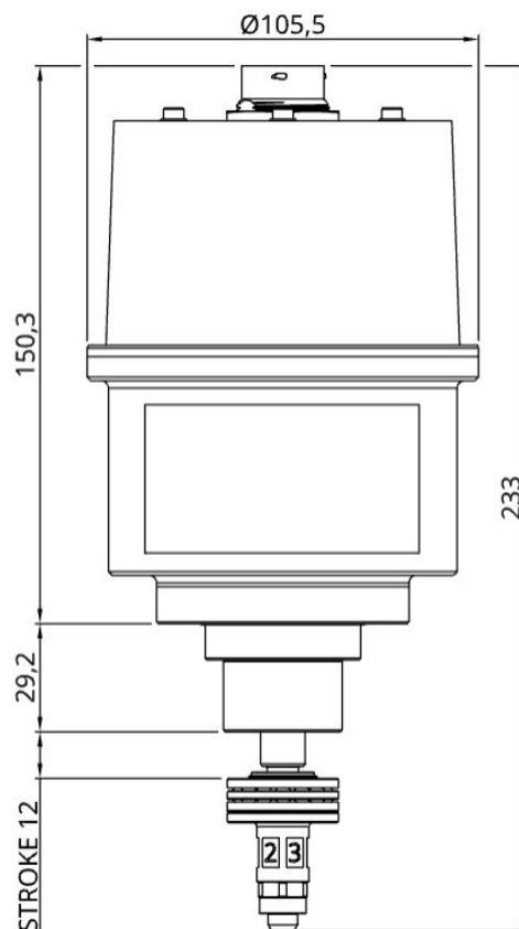
SB750 Actuator 0800-000132
